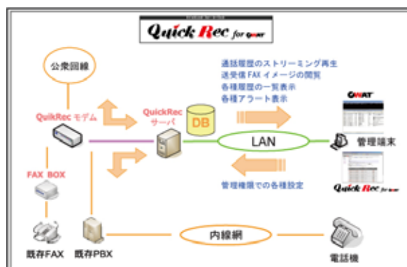
【QuickRec for CWAT構成概要図】
